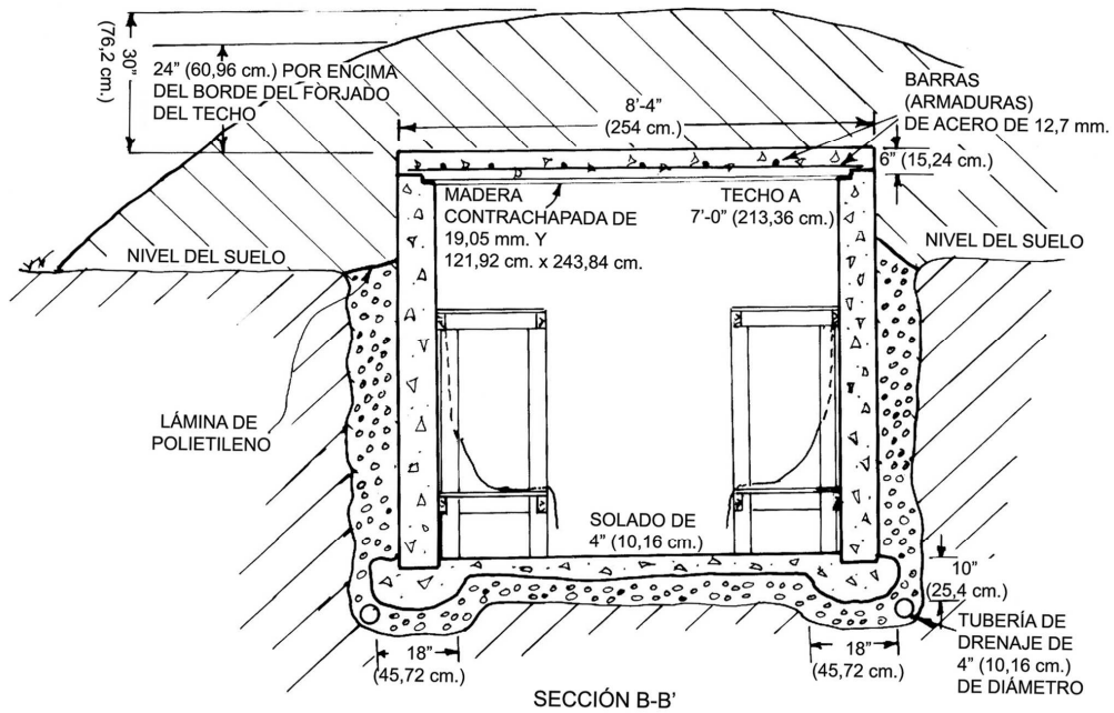
SECCIÓN B-B'
