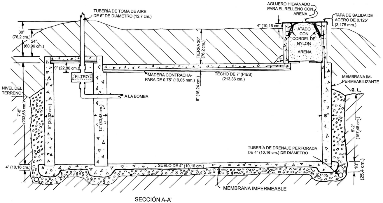
SECCIÓN A-A'
